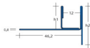
Ausführung links
