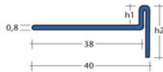
Ausführung links
