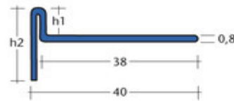
Ausführung rechts
